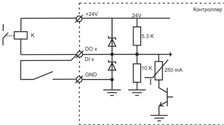
Рисунок 6.9- Универсальный дискретный выход/вход типа DODI24U
